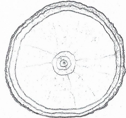
rodochrozyt
