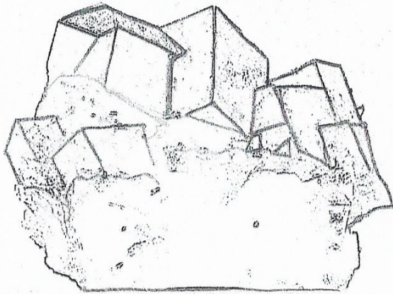
fluoryt
