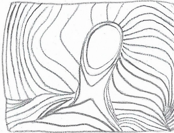
krzemien pasiasty
